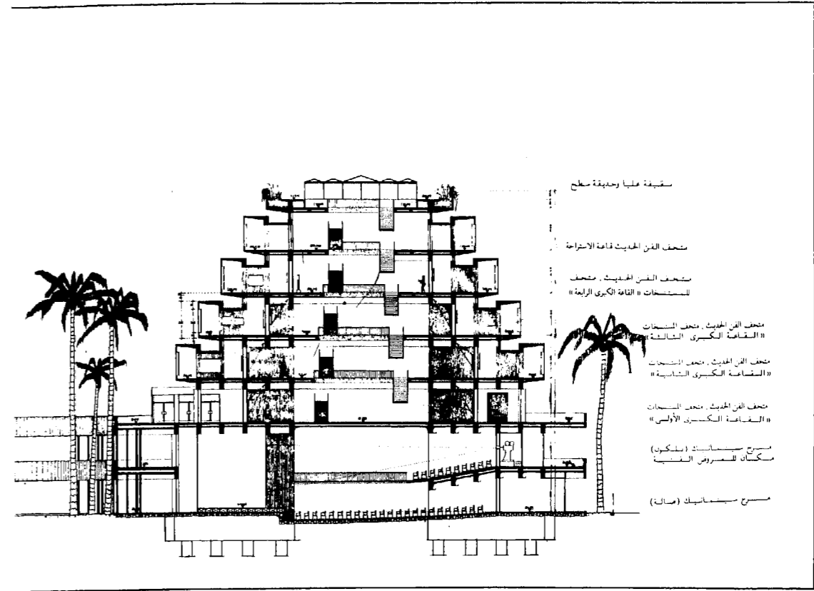
قصر الفنون : قطاع طولي للمبنى الشرقي والمبنى الغربي.
